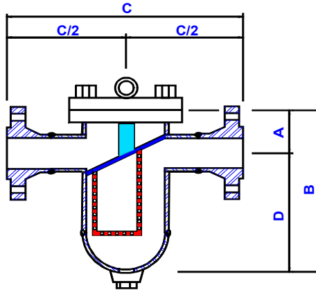
SHOWN WITH OPTIONAL LIFT LUG
